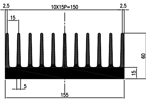
F60155R 11.31Kg/m
