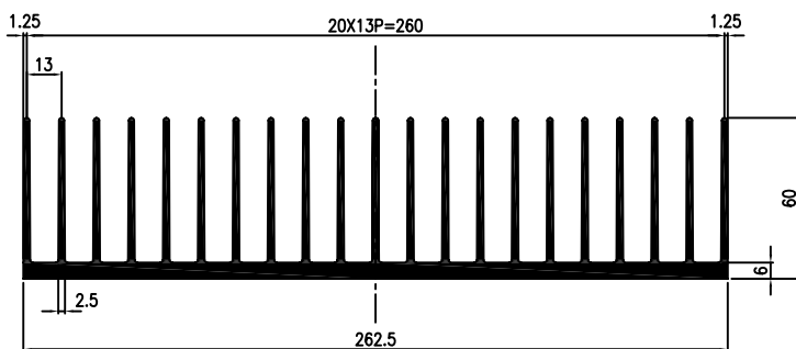
F60262 11.1Kg/m
