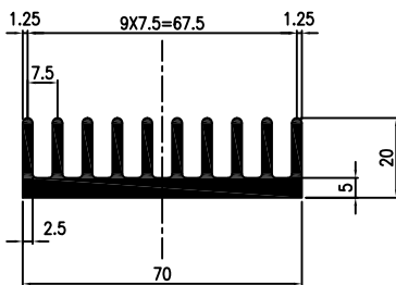
F2070 1.95Kg/m
