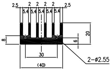
F2040H 1.16Kg/m
