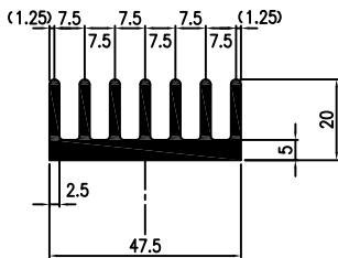
F2047 1.34Kg/m
