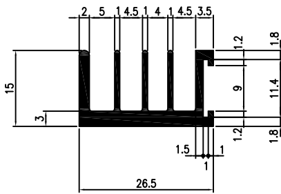
基板推奨穴径 \phi 2.3
